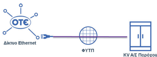
Εικόνα 5: Σχηματική απεικόνιση πρόσβασης Ethernet από Καμπίνα Απομακρυσμένης Συνεγκατάστασης
